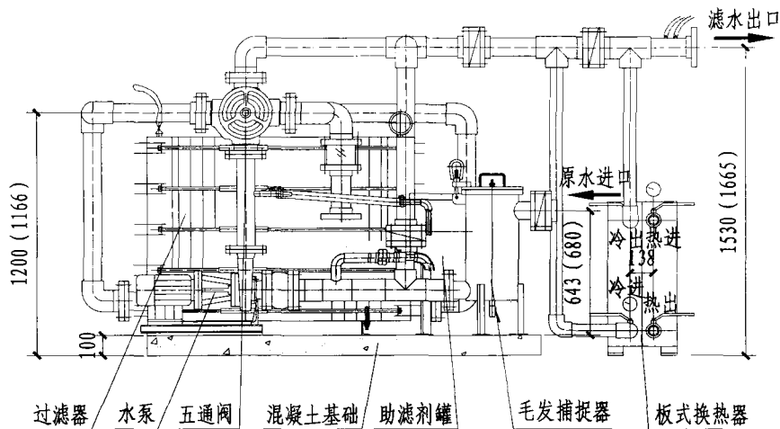
立面图
