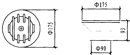
SP-1424B池壁进水口
