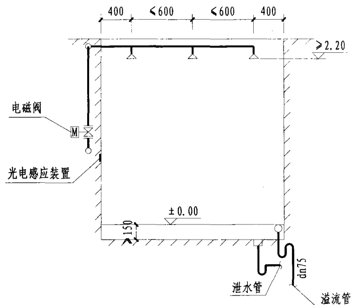
A-A剖面图
