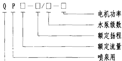
水泵型号标注示意
