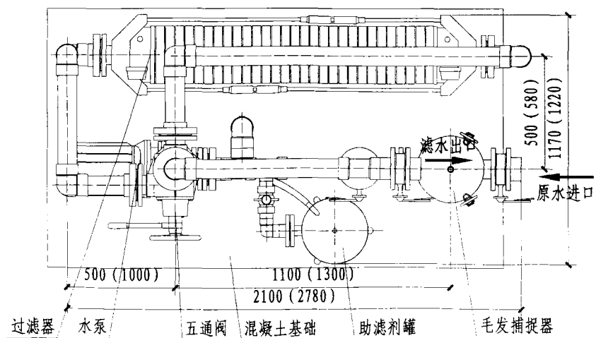
立面图
