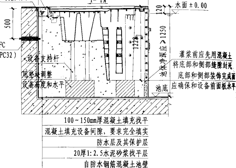
A-A 剖面图
