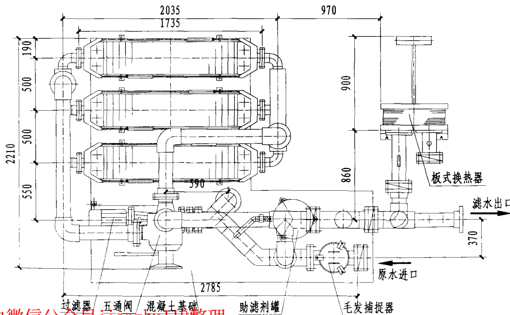
平面图
