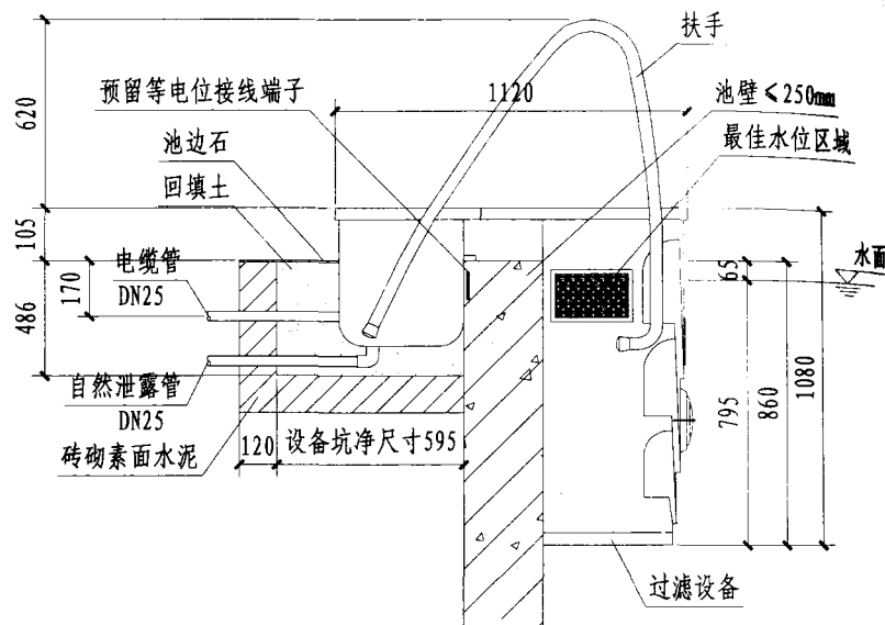
A-A 剖面图
