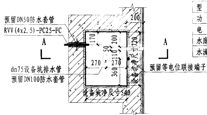
设备坑平面图
