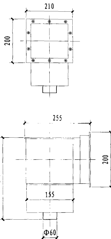
WL-APZ02标准撇沫器
