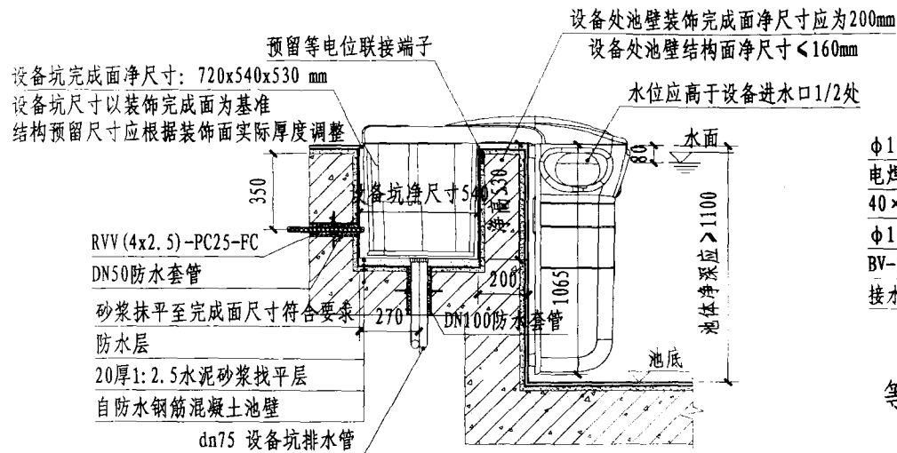
A-A 剖面图
