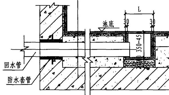
回水口安装 (b)
