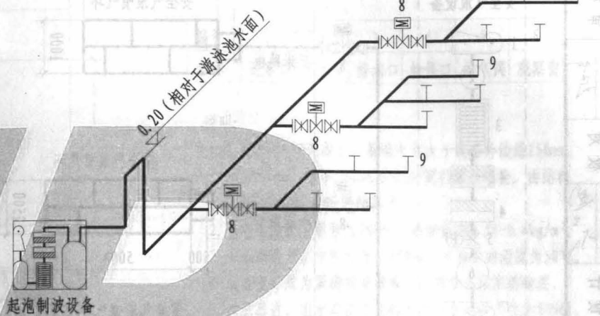
跳台或跳板前方局部制波系统图
