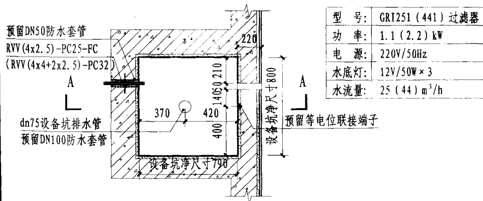
设备坑平面图
