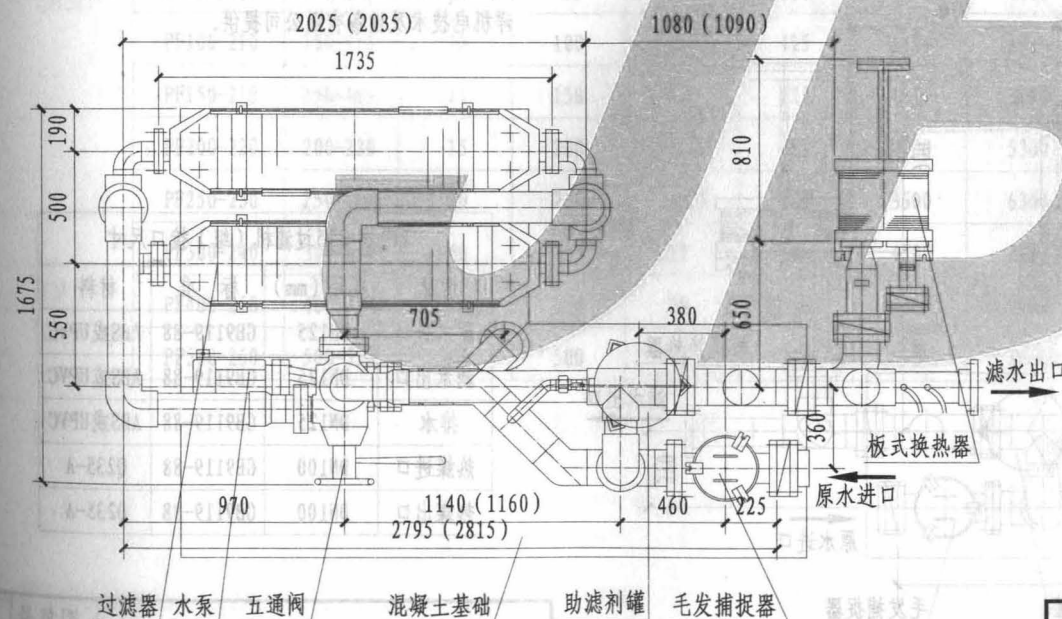
立面图
