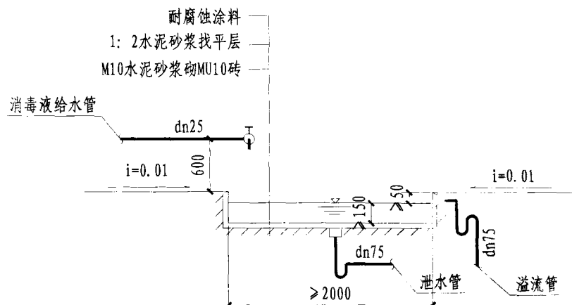
A-A浸脚消毒池剖面图
